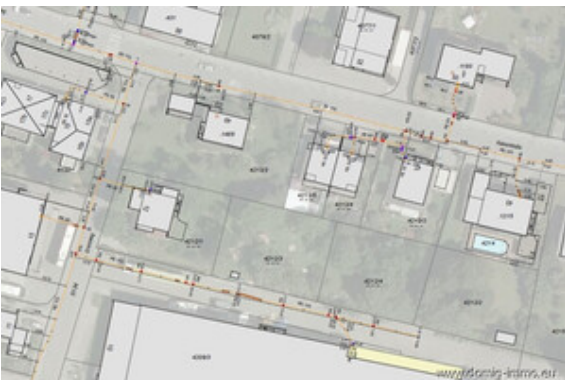
Gasleitung
